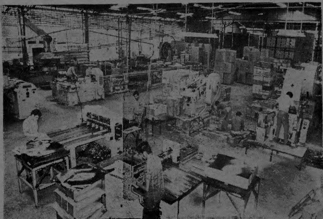
FABRICA DE ENVASES - Vista panorámica de maquinaria para cortar la hojalata y para Estampado de TAPAS Y FONDOS. En segundo término, maquinaria para hacer cuerpos de envases.
